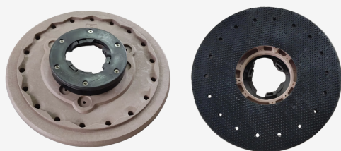
1 disco portapad
